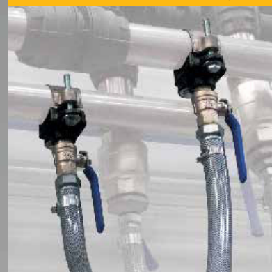
Anschlussleitung
