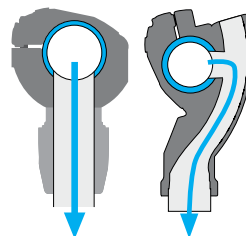
Vertikaler Abgang
